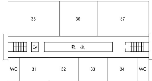
〔 3 階 〕
