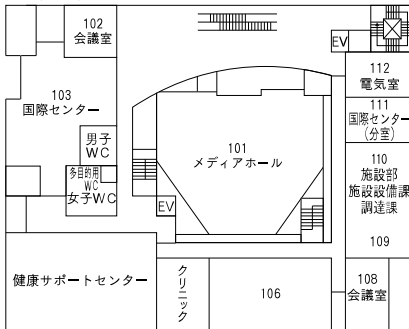
〔1階〕
